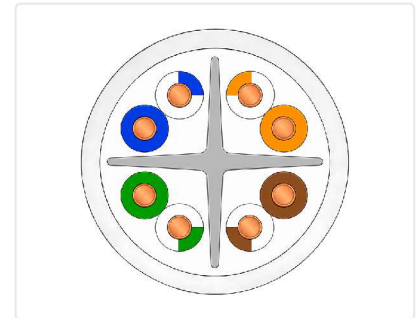
CORTE TRANSVERSAL
