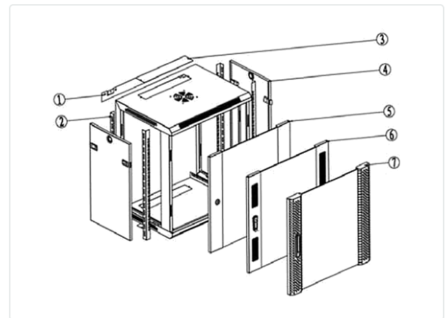
DESPIECE · DIBUJO DEL FABRICANTE
