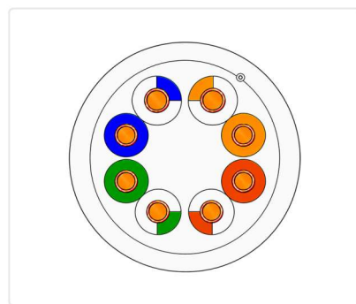
CORTE TRANSVERSAL
