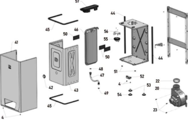
Cuerpo caldera
