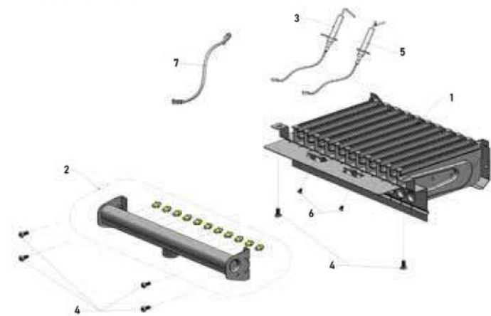
Grupo Quemador
