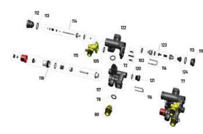
Grupo Quemador
