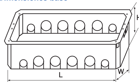
Dimensiones base
