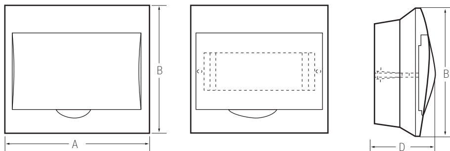
Dimensiones tapa
