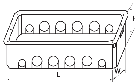
Dimensiones base
