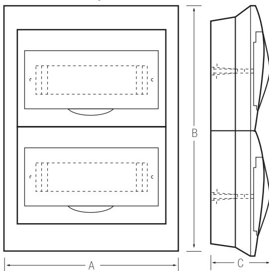
Dimensiones tapa
