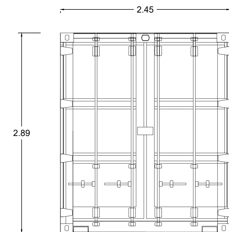
Elevación (D)
