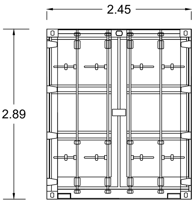
Elevación (D)
