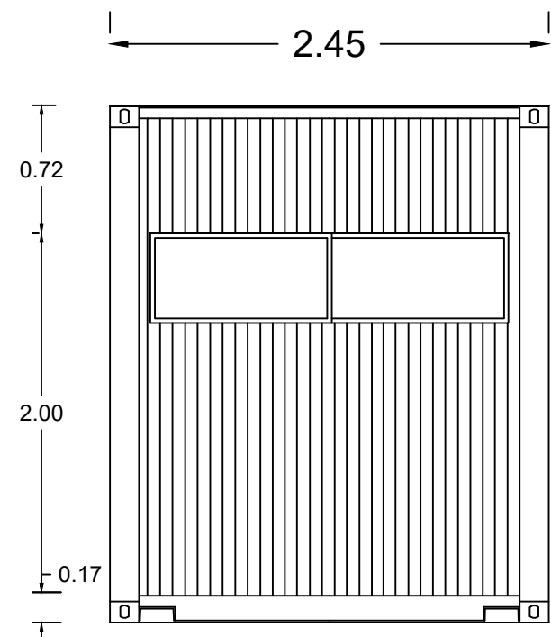
Elevación (B)
