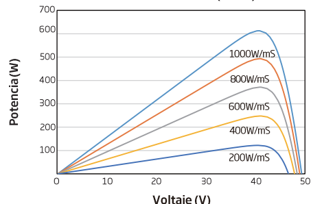
CURVAS P-V DEL MÓDULO (615W)
