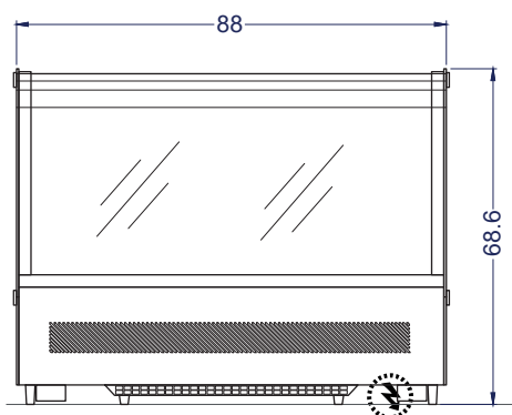
Vista Elevación
