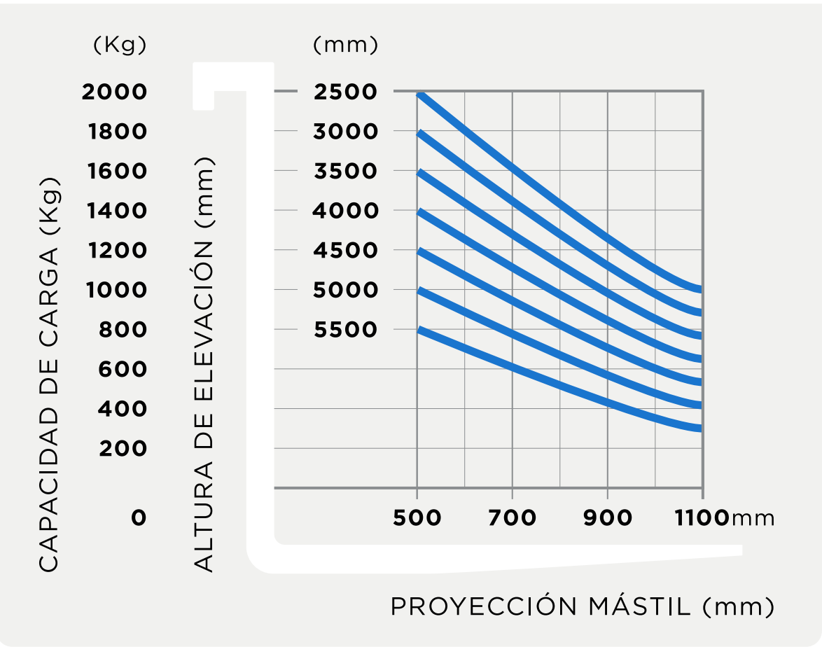
GRÁFICO DE CARGA
