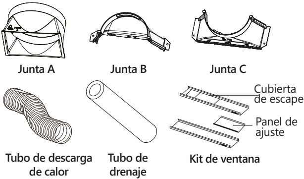
Accesorios e instalación de la manguera de escape de calor.
