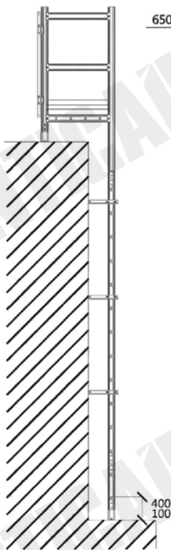
VISTA LATERAL
