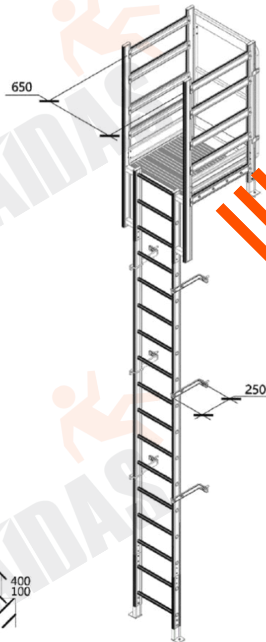
VISTA ISOMÉTRICA
