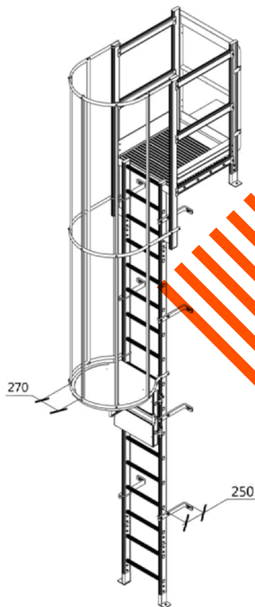
VISTA ISOMÉTRICA
